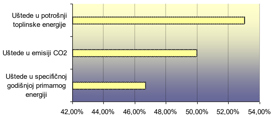
Graf br. 1. Uštede u okviru energetske obnove OŠ I.G.Kovačića Gornje Bazje
