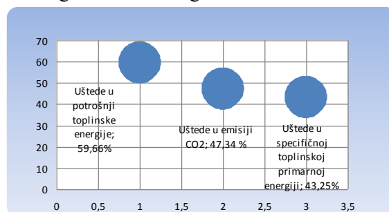
Uštede u okviru energetske obnove zgrade B OŠ Petra Preradovića Pitomača
