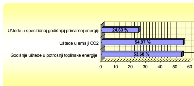
Grafički prikaz br. 4. Uštede u okviru energetske obnove zgrade dvorane Tehničke škole Virovitica
