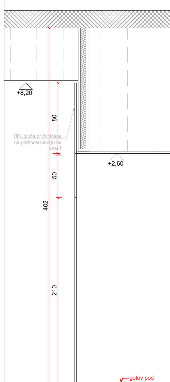
PRESJEK A-A
